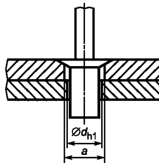
Рисунок 2 — Увеличенный диаметр отверстия для облегчения совмещения
