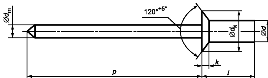
Рисунок 1 — Размеры заклепок
